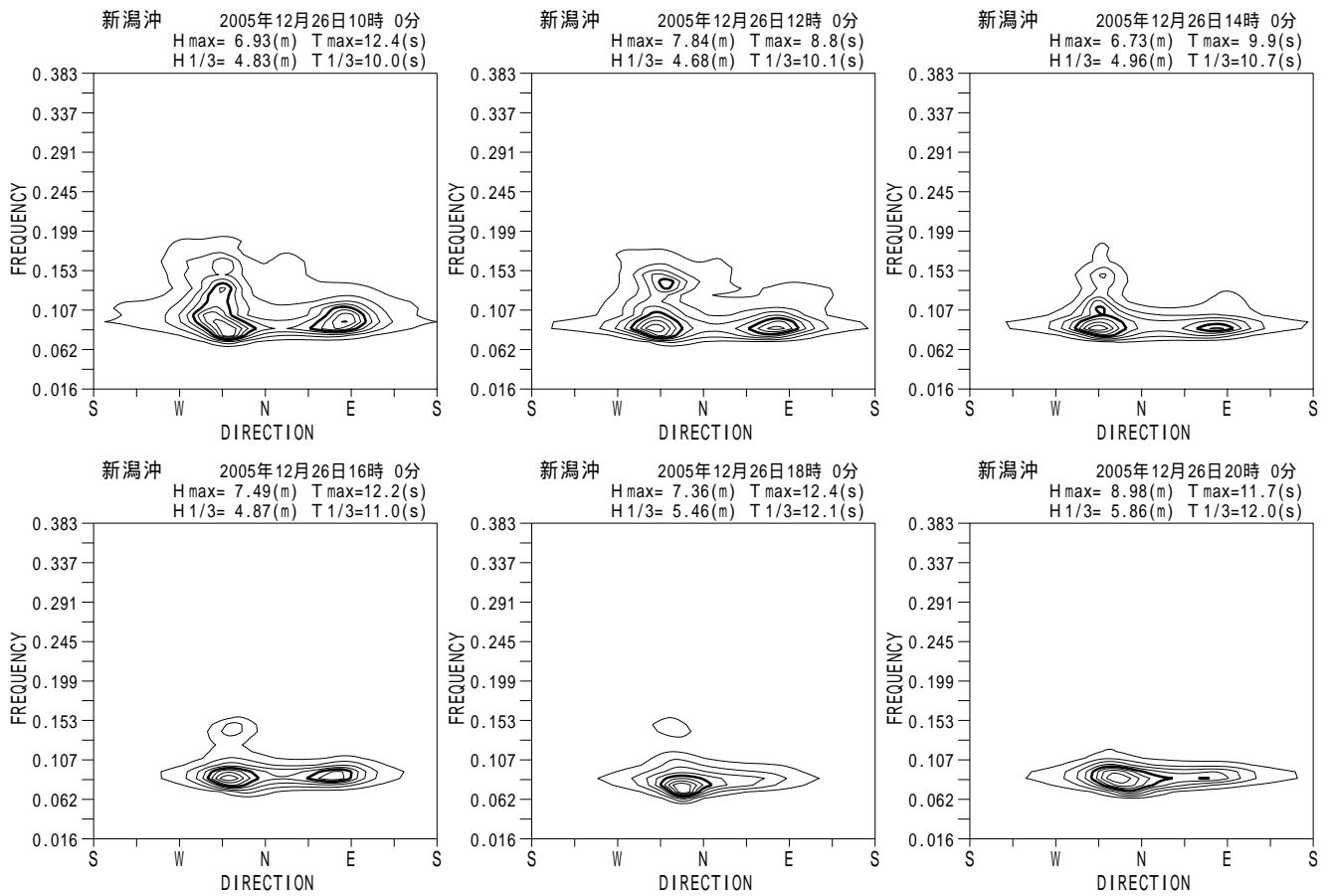
付図 - A.5.7 新潟沖 代表的な高波期間中の方向スペクトル
