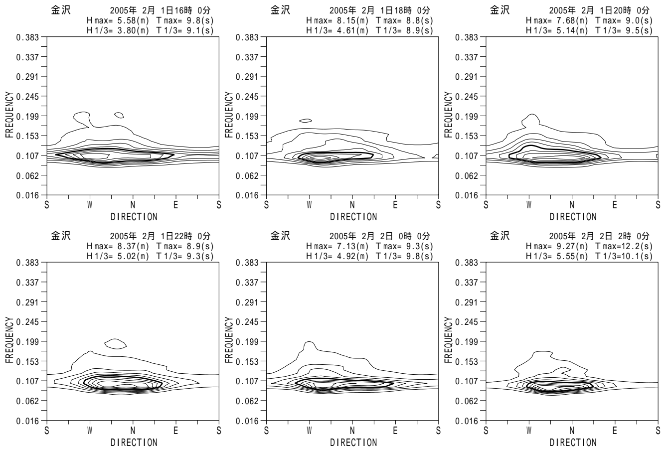
付図 - A.5.12 金沢 代表的な高波期間中の方向スペクトル
