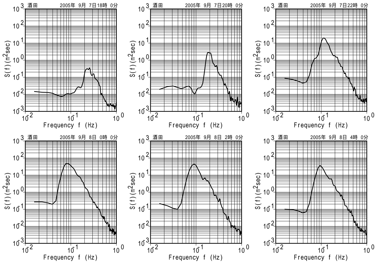
付図 - A.5.6 酒田 代表的な高波期間中のスペクトル
