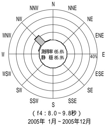
付図 - B.4.61 石垣沖 波高・波向別出現頻度図 ( 連続観測 , f2 , f3 , f4 , f5 , 全周期帯 )
