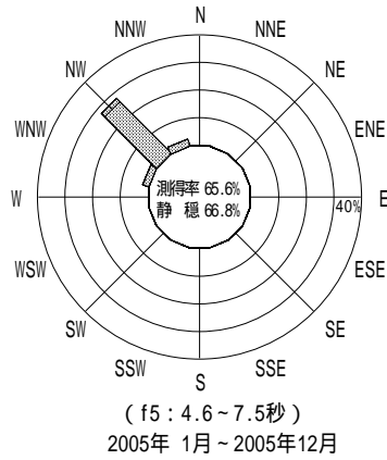
付図 - B.4.61 石垣沖 波高・波向別出現頻度図 ( 連続観測 , f2 , f3 , f4 , f5 , 全周期帯 )
