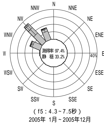
付図 - B.4.2 石狩新港 波高・波向別出現頻度図 ( 連続観測 , f2 , f3 , f4 , f5 , 全周期帯 )
