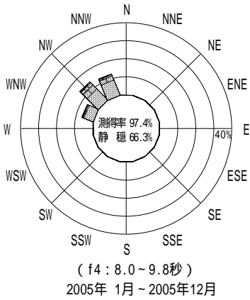
付図 - B.4.2 石狩新港 波高・波向別出現頻度図 ( 連続観測 , f2 , f3 , f4 , f5 , 全周期帯 )
