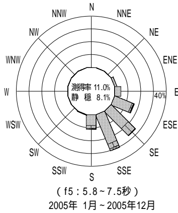
付図 - B.4.54 細島 波高・波向別出現頻度図 ( 連続観測 , f2 , f3 , f4 , f5 , 全周期帯 )
