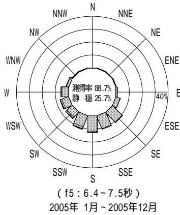
付図 - B.4.46 潮岬 波高・波向別出現頻度図 (連続観測, f2, f3, f4, f5, 全周期帯)
