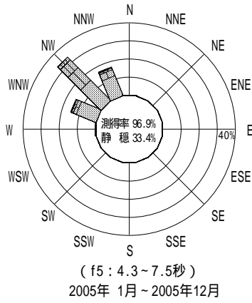
付図 - A.4.2 石狩新港 波高・波向別出現頻度図 ( f2 , f3 , f4 , f5 , 全周期帯 )
