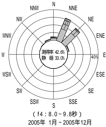
付図 - A.4.25 紋別(南) 波高・波向別出現頻度図 ( f2 , f3 , f4 , f5 , 全周期帯 )
