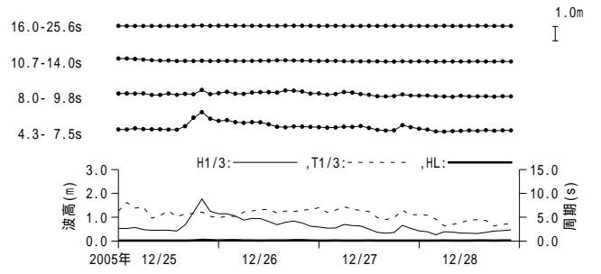
付図 - A.3.40 アシカ島 周期帯別波浪特性の経時変化(高波期間中)
