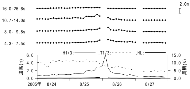
付図 - A.3.40 アシカ島 周期帯別波浪特性の経時変化(高波期間中)
