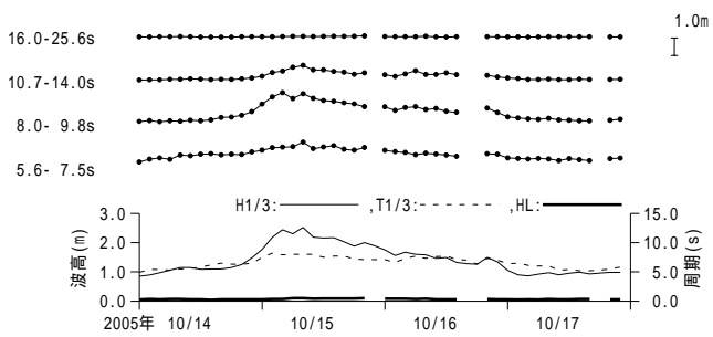
付図 - A.3.59 平良沖 周期帯別波浪特性の経時変化(高波期間中)
