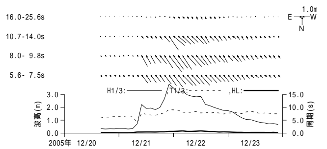
付図 - A.3.59 平良沖 周期帯別波浪特性の経時変化(高波期間中)
