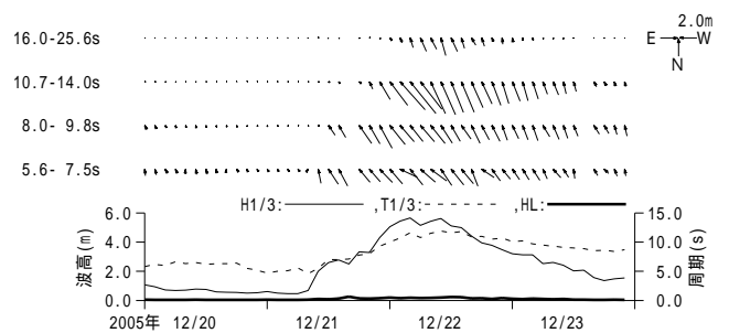
付図 - A.3.24 那覇 周期帯別波浪特性の経時変化(高波期間中)
