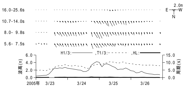
付図 - A.3.24 那覇 周期帯別波浪特性の経時変化(高波期間中)
