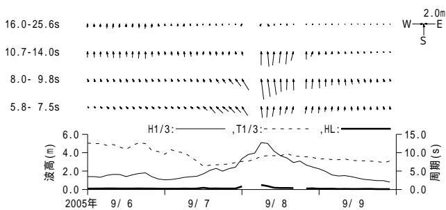
付図 - A.3.26 釧路 周期帯別波浪特性の経時変化(高波期間中)
