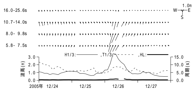
付図 - A.3.26 釧路 周期帯別波浪特性の経時変化(高波期間中)
