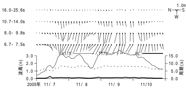
付図 - A.3.3 瀬棚 周期帯別波浪特性の経時変化(高波期間中)
