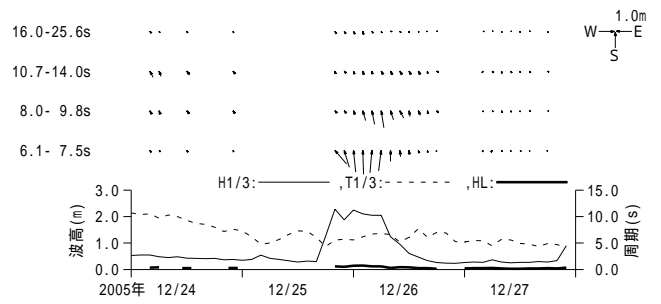
付図 - A.3.28 苫小牧 周期帯別波浪特性の経時変化(高波期間中)
