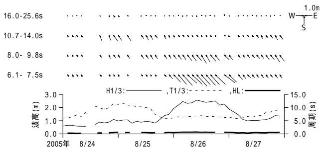
付図 - A.3.28 苫小牧 周期帯別波浪特性の経時変化(高波期間中)
