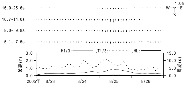
付図 - A.3.45 伊勢湾 周期帯別波浪特性の経時変化(高波期間中)
