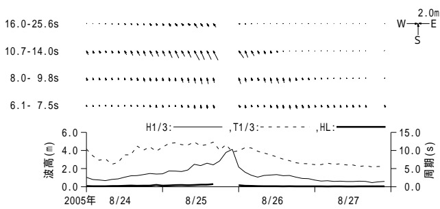
付図 - A.3.43 清水 周期帯別波浪特性の経時変化(高波期間中)
