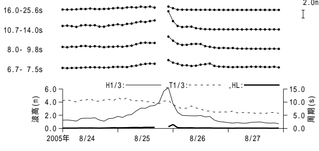
付図 - A.3.42 下田 周期帯別波浪特性の経時変化(高波期間中)
