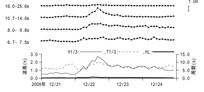
付図 - A.3.42 下田 周期帯別波浪特性の経時変化(高波期間中)
