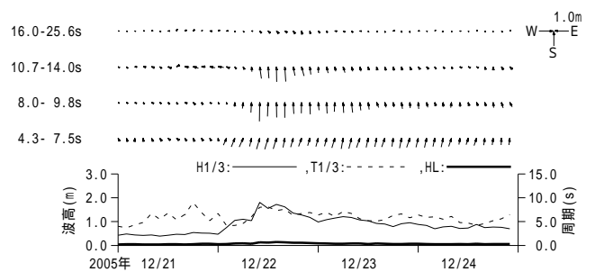
付図 - A.3.44 御前崎 周期帯別波浪特性の経時変化(高波期間中)
