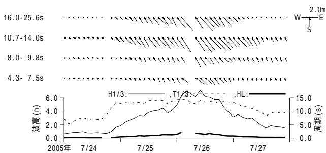
付図 - A.3.44 御前崎 周期帯別波浪特性の経時変化(高波期間中)
