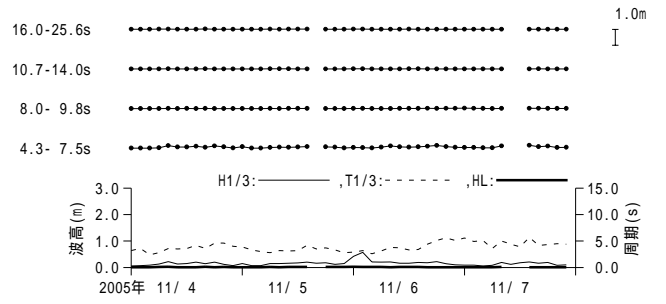
付図 - A.3.56 鹿児島 周期帯別波浪特性の経時変化(高波期間中)
