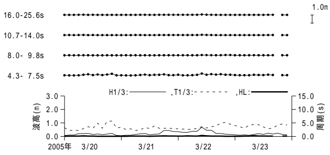
付図 - A.3.56 鹿児島 周期帯別波浪特性の経時変化(高波期間中)
