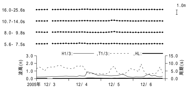
付図 - A.3.55 志布志湾 周期帯別波浪特性の経時変化(高波期間中)
