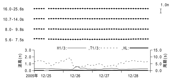
付図 - A.3.55 志布志湾 周期帯別波浪特性の経時変化(高波期間中)
