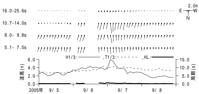
付図 - A.3.21 玄界灘 周期帯別波浪特性の経時変化(高波期間中)
