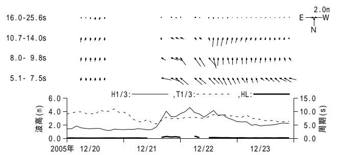
付図 - A.3.21 玄界灘 周期帯別波浪特性の経時変化(高波期間中)
