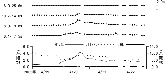
付図 - A.3.49 室戸GPS 周期帯別波浪特性の経時変化(高波期間中)
