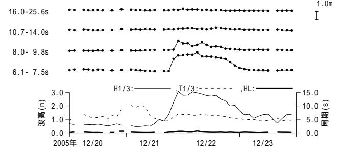
付図 - A.3.49 室戸GPS 周期帯別波浪特性の経時変化(高波期間中)
