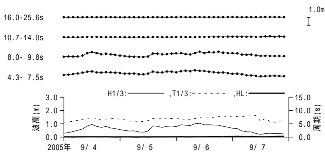
付図 - A.3.16 柴山(港内) 周期帯別波浪特性の経時変化(高波期間中)
