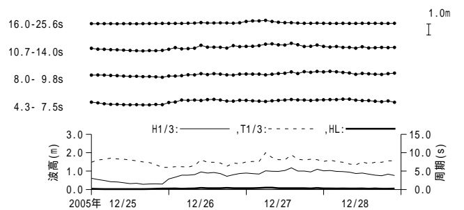
付図 - A.3.16 柴山(港内) 周期帯別波浪特性の経時変化(高波期間中)
