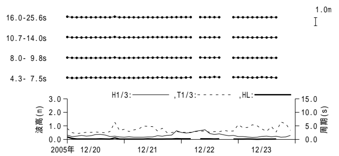
付図 - A.3.48 小松島 周期帯別波浪特性の経時変化(高波期間中)
