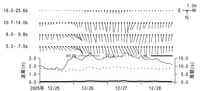
付図 - A.3.15 柴山 周期帯別波浪特性の経時変化(高波期間中)
