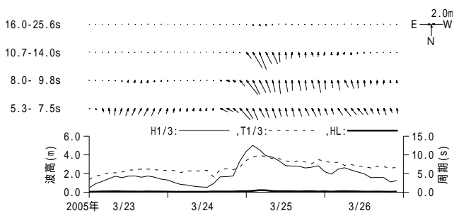
付図 - A.3.15 柴山 周期帯別波浪特性の経時変化(高波期間中)
