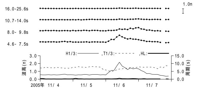
付図 - A.3.52 上川口 周期帯別波浪特性の経時変化(高波期間中)
