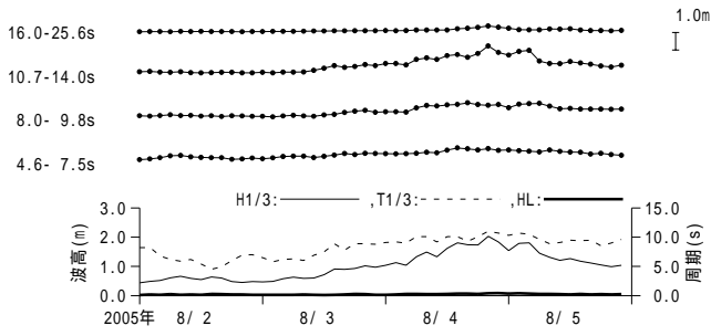
付図 - A.3.52 上川口 周期帯別波浪特性の経時変化(高波期間中)
