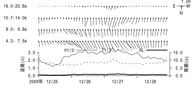
付図 - A.3.17 鳥取 周期帯別波浪特性の経時変化(高波期間中)
