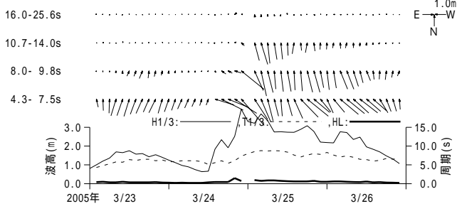
付図 - A.3.17 鳥取 周期帯別波浪特性の経時変化(高波期間中)
