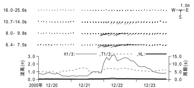
付図 - A.3.46 潮岬 周期帯別波浪特性の経時変化(高波期間中)
