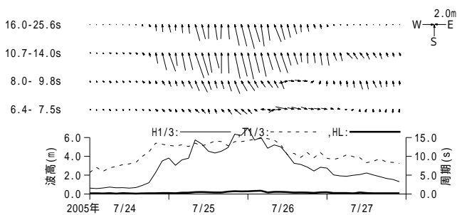
付図 - A.3.46 潮岬 周期帯別波浪特性の経時変化(高波期間中)
