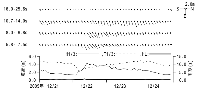
付図 - A.3.31 久慈 周期帯別波浪特性の経時変化(高波期間中)
