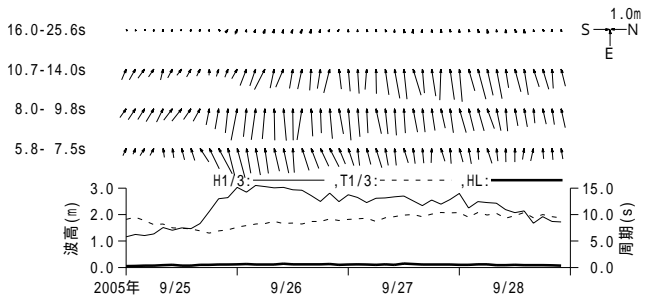
付図 - A.3.31 久慈 周期帯別波浪特性の経時変化(高波期間中)
