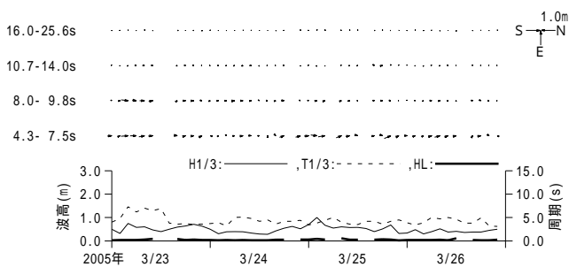
付図 - A.3.39 第二海堡 周期帯別波浪特性の経時変化(高波期間中)
