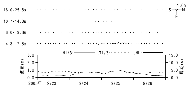
付図 - A.3.39 第二海堡 周期帯別波浪特性の経時変化(高波期間中)
