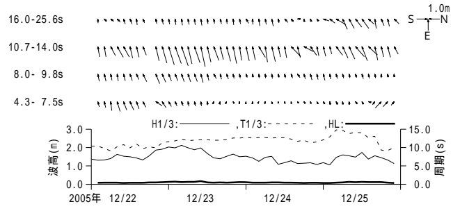
付図 - A.3.35 相馬 周期帯別波浪特性の経時変化(高波期間中)
