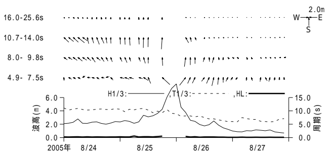
付図 - A.3.41 波浮 周期帯別波浪特性の経時変化(高波期間中)
