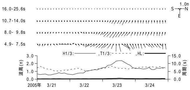
付図 - A.3.37 常陸那珂 周期帯別波浪特性の経時変化(高波期間中)
