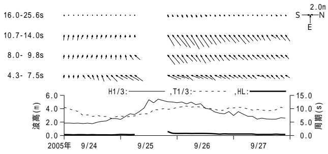
付図 - A.3.38 鹿島 周期帯別波浪特性の経時変化(高波期間中)
