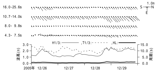
付図 - A.3.38 鹿島 周期帯別波浪特性の経時変化(高波期間中)
