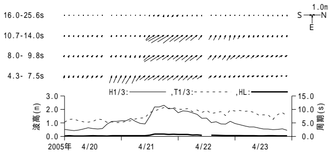
付図 - A.3.34 仙台新港 周期帯別波浪特性の経時変化(高波期間中)
