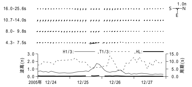
付図 - A.3.34 仙台新港 周期帯別波浪特性の経時変化(高波期間中)
