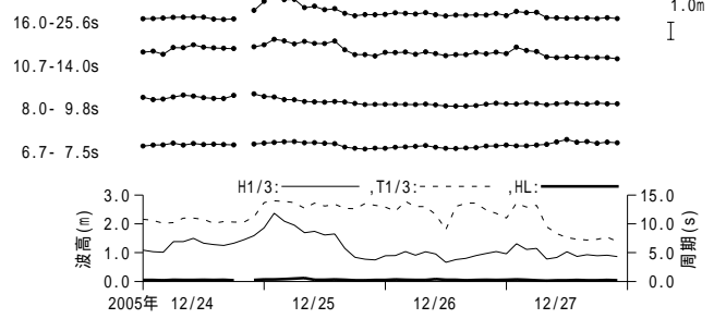
付図 - A.3.32 釜石 周期帯別波浪特性の経時変化(高波期間中)
