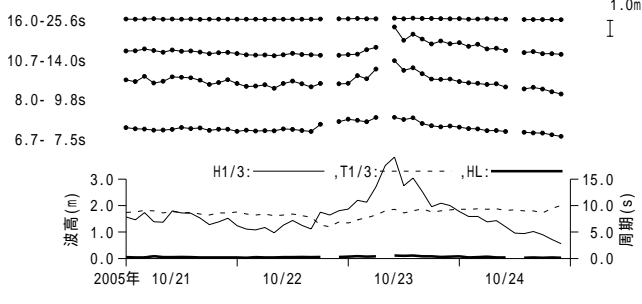
付図 - A.3.32 釜石 周期帯別波浪特性の経時変化(高波期間中)
