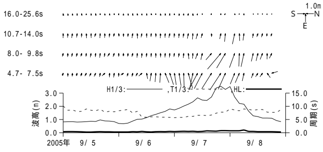
付図 - A.3.29 むつ小川原 周期帯別波浪特性の経時変化(高波期間中)
