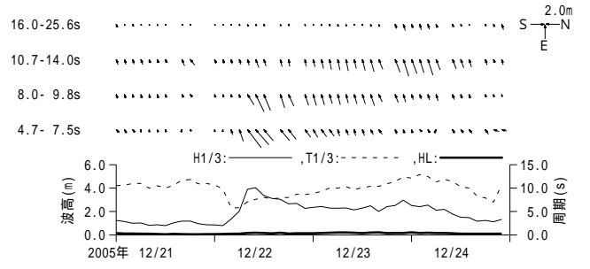
付図 - A.3.29 むつ小川原 周期帯別波浪特性の経時変化(高波期間中)
