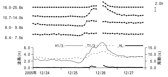
付図 - A.3.4 深浦 周期帯別波浪特性の経時変化(高波期間中)
