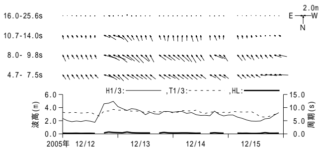
付図 - A.3.13 福井 周期帯別波浪特性の経時変化(高波期間中)
