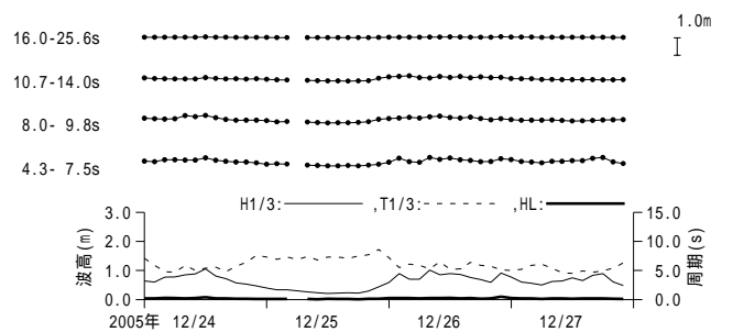
付図 - A.3.14 敦賀 周期帯別波浪特性の経時変化(高波期間中)
