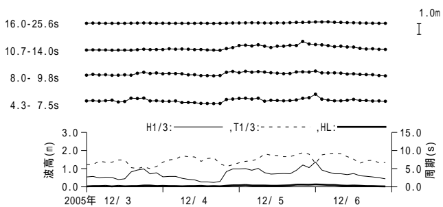
付図 - A.3.14 敦賀 周期帯別波浪特性の経時変化(高波期間中)
