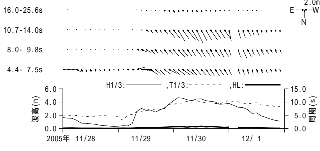
付図 - A.3.8 直江津 周期帯別波浪特性の経時変化(高波期間中)
