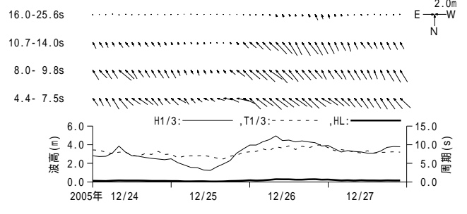
付図 - A.3.8 直江津 周期帯別波浪特性の経時変化(高波期間中)
