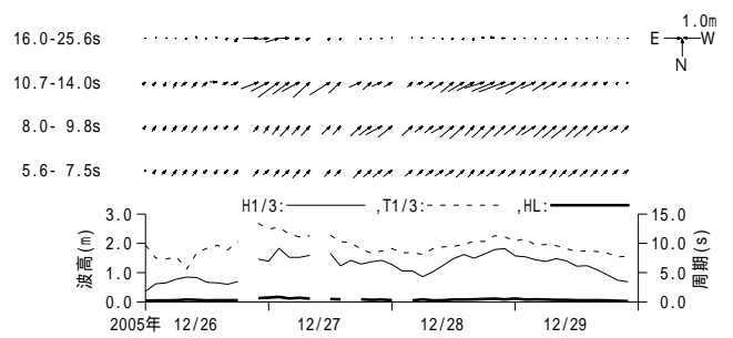
付図 - A.3.10 伏木富山 周期帯別波浪特性の経時変化(高波期間中)
