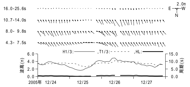
付図 - A.3.12 金沢 周期帯別波浪特性の経時変化(高波期間中)
