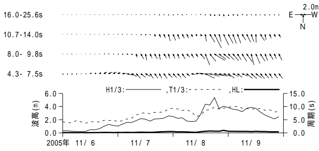
付図 - A.3.12 金沢 周期帯別波浪特性の経時変化(高波期間中)
