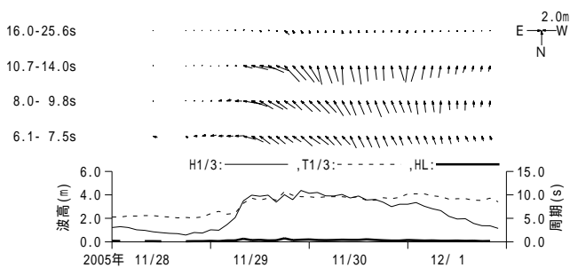
付図 - A.3.11 輪島 周期帯別波浪特性の経時変化(高波期間中)
