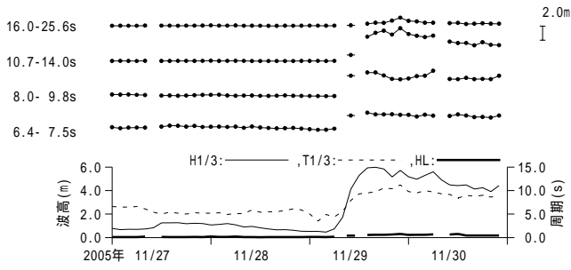
付図 - A.3.6 酒田 周期帯別波浪特性の経時変化(高波期間中)
