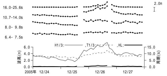
付図 - A.3.6 酒田 周期帯別波浪特性の経時変化(高波期間中)
