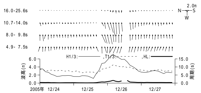
付図 - A.3.5 秋田 周期帯別波浪特性の経時変化(高波期間中)
