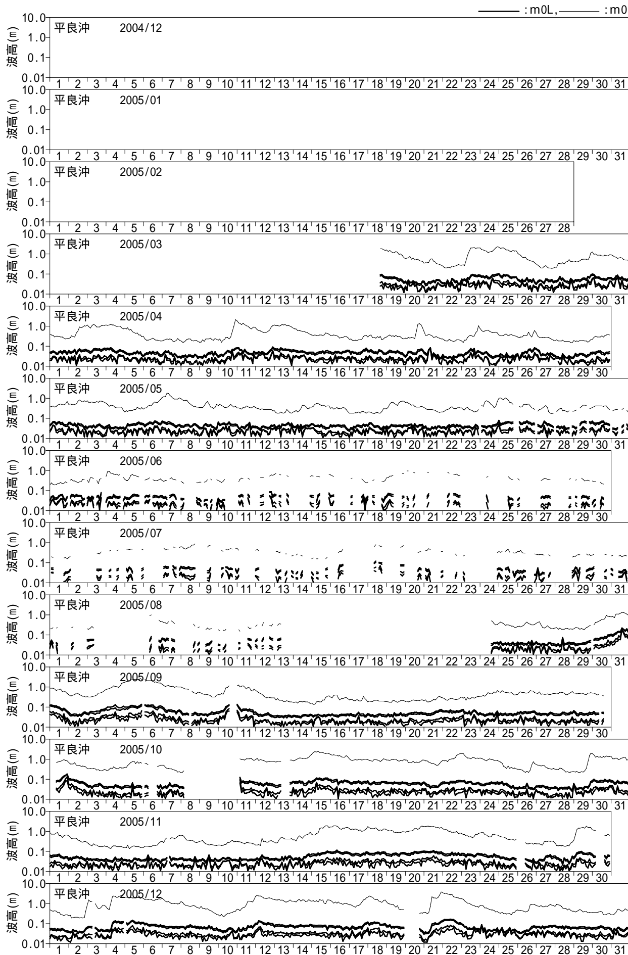
付図 - C.1.59 長周期波高の経時変化図 (平良沖)
