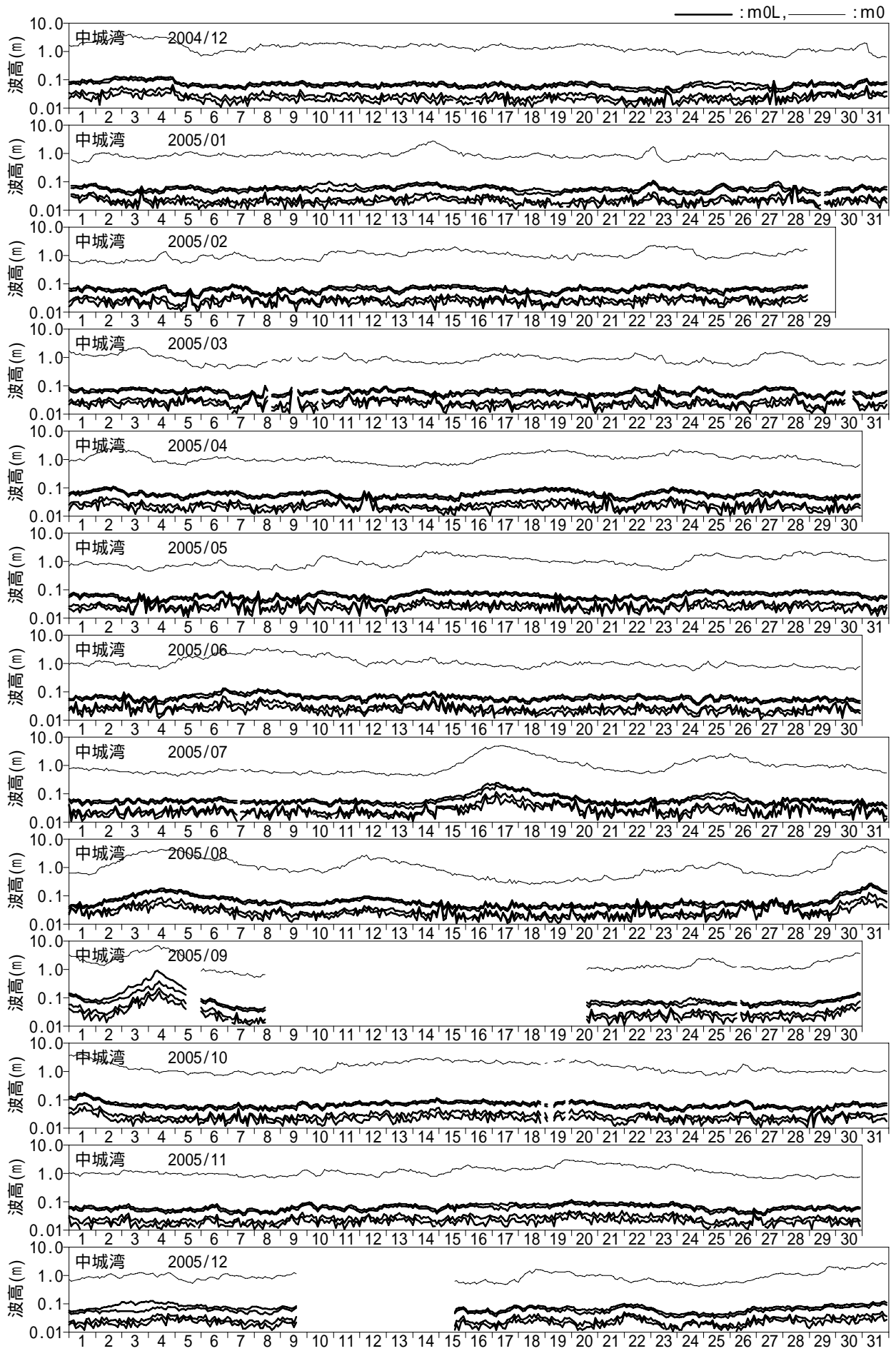
付図 - C.1.57 長周期波高の経時変化図 (中城湾)
