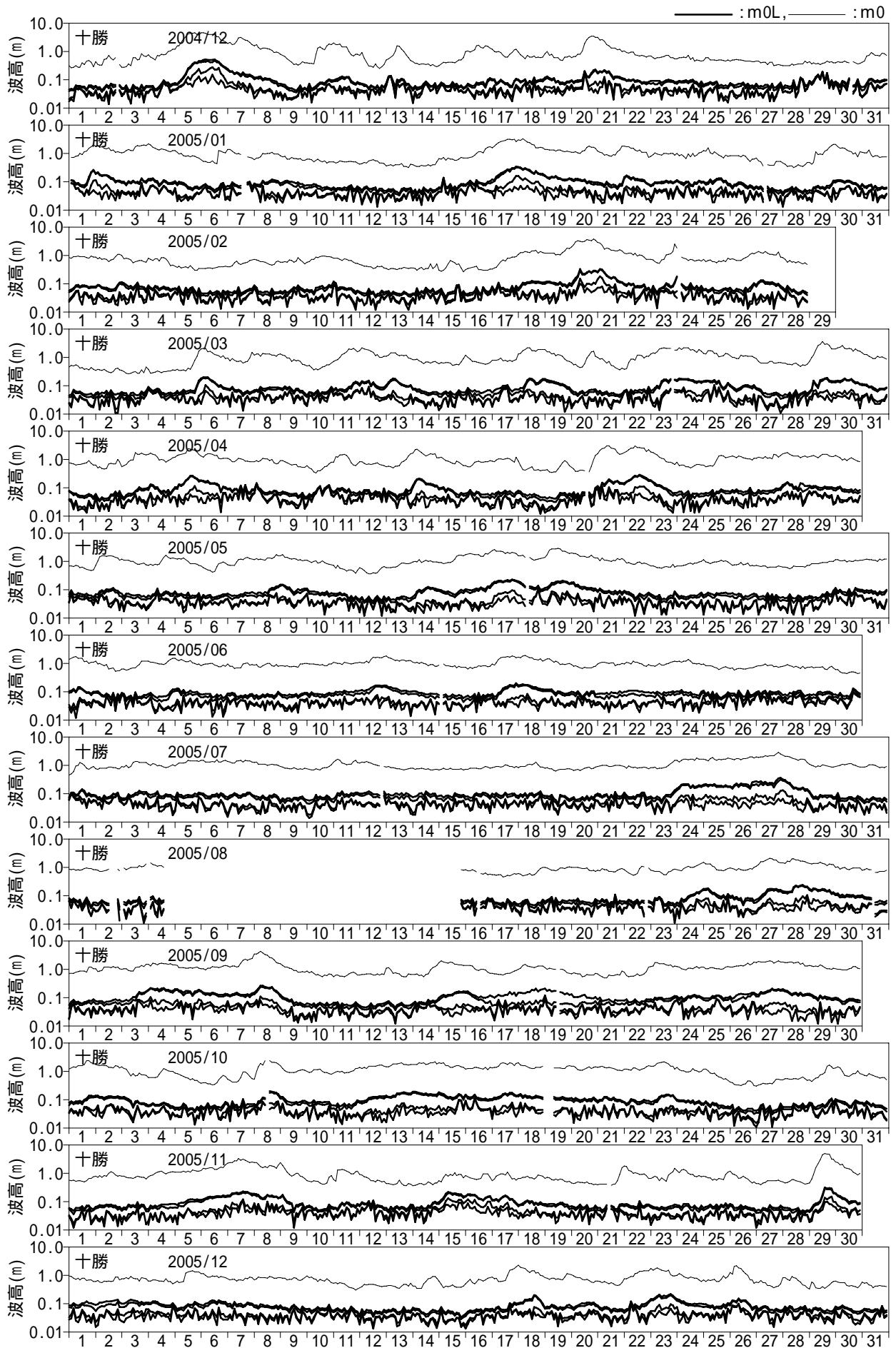
付図 - C.1.27 長周期波高の経時変化図 (十勝)
